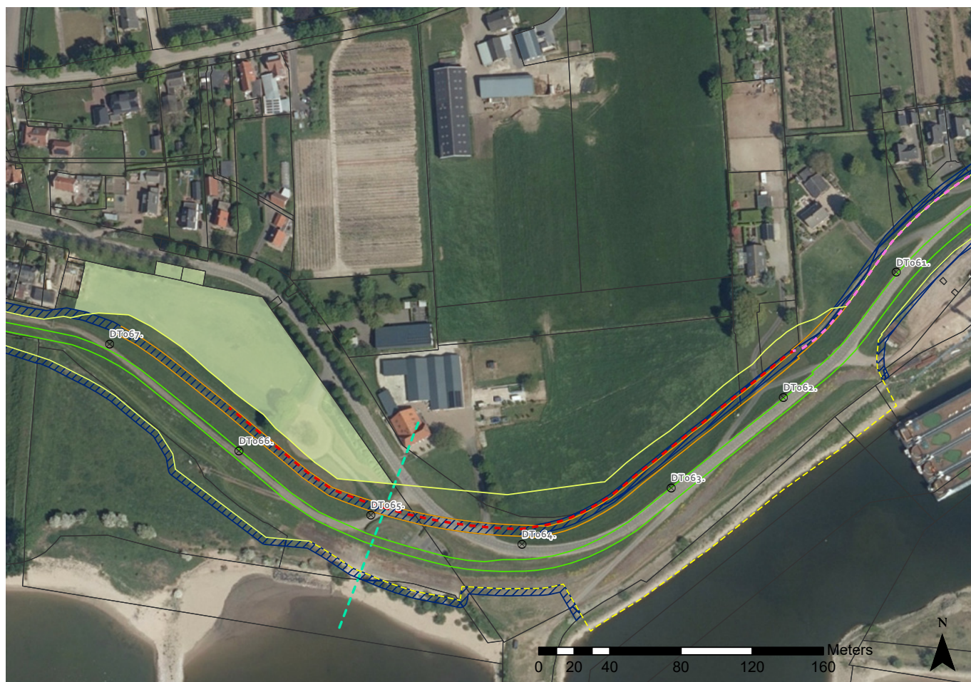
Figuur 2.12 Ontwerp dijkversterking traject De Snor DT062-DT066+050
