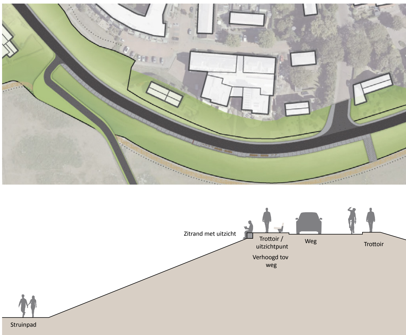
Figuur 3.1 Inpassingen bij dorpsfront Ochten
