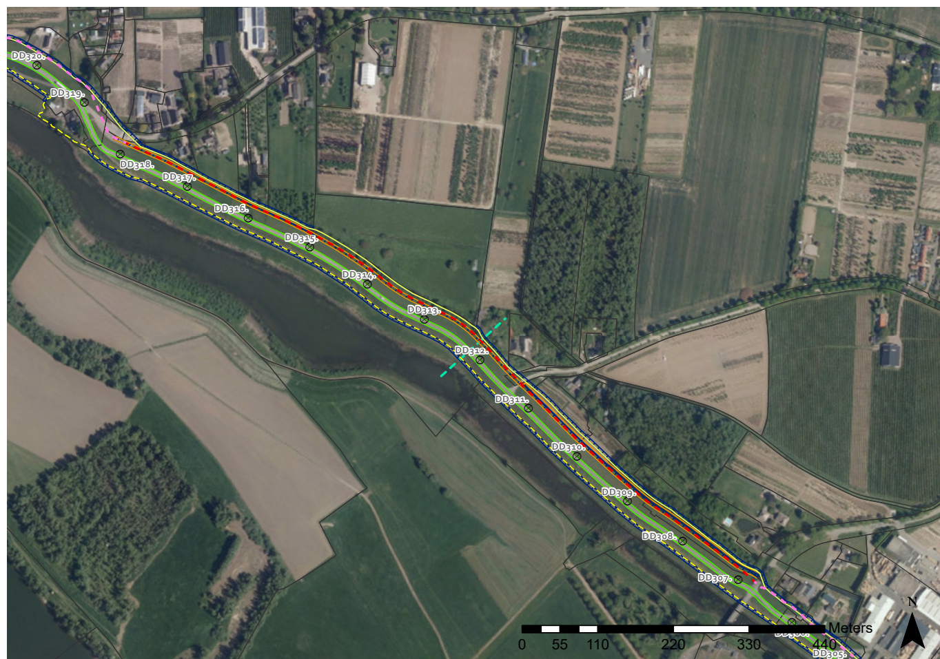
Figuur 2.8 Ontwerp dijkversterking traject Dodewaard DD307-DD318
